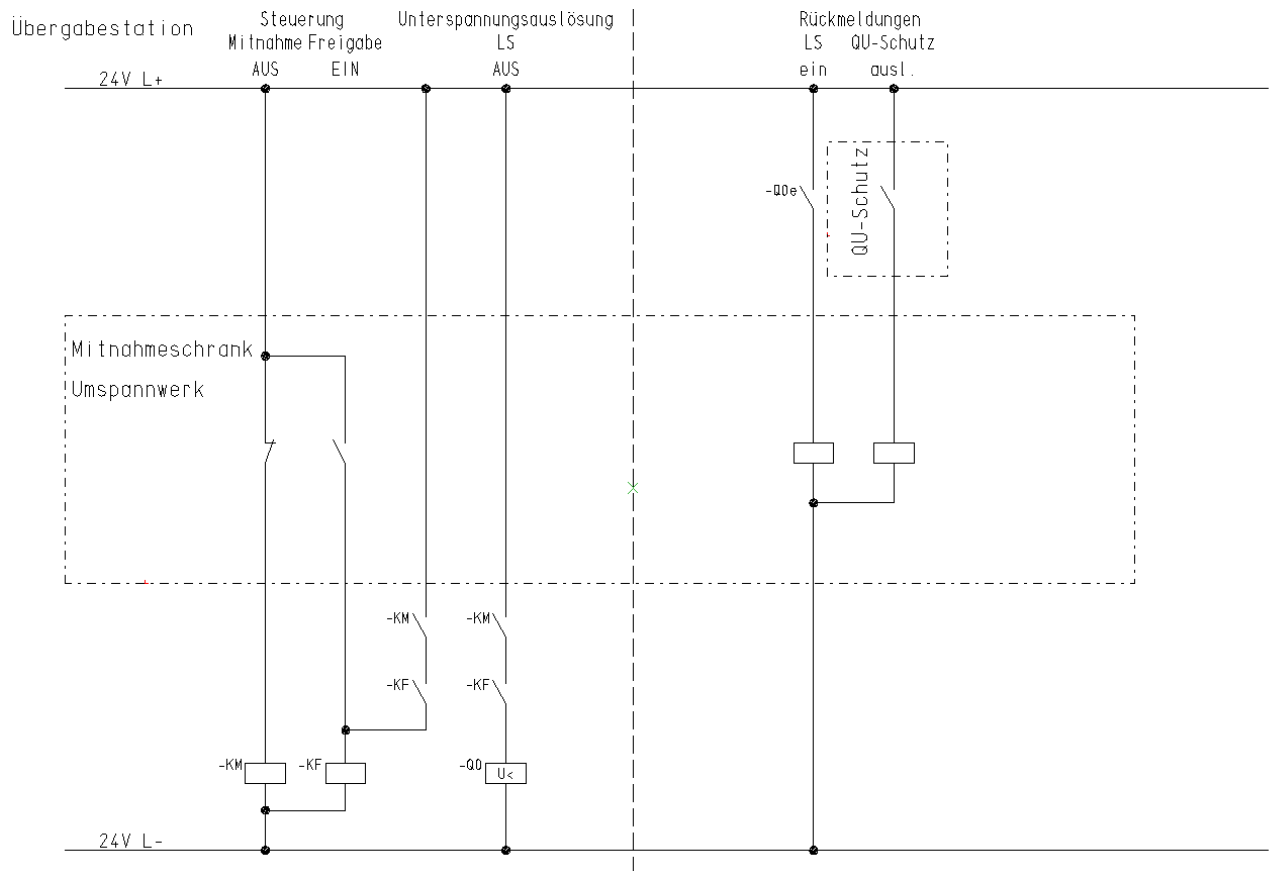
Schaltungsaufbau der Steuerkabelverbindung zwischen der Übergabestation und dem Westnetz-eigenen Umspannwerk
